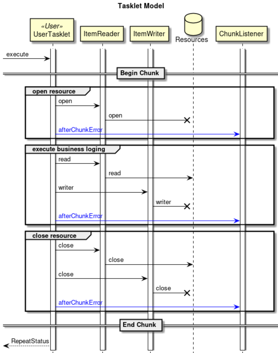
図 45. タスケレットモデルでの例外ハンドリング概略図
