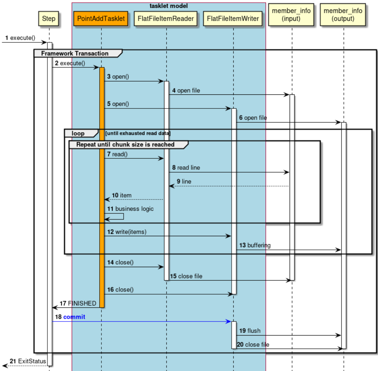
図 87. タスクレットモデルのシーケンス図
