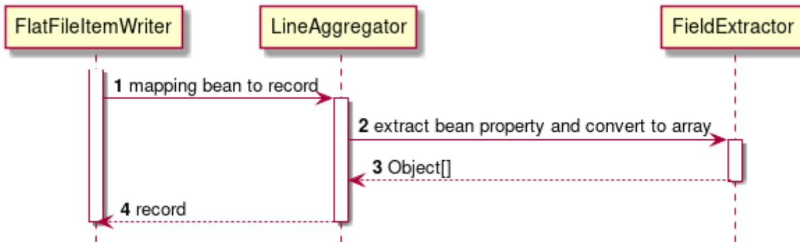
図 39. 各コンポーネントの呼び出し関係
