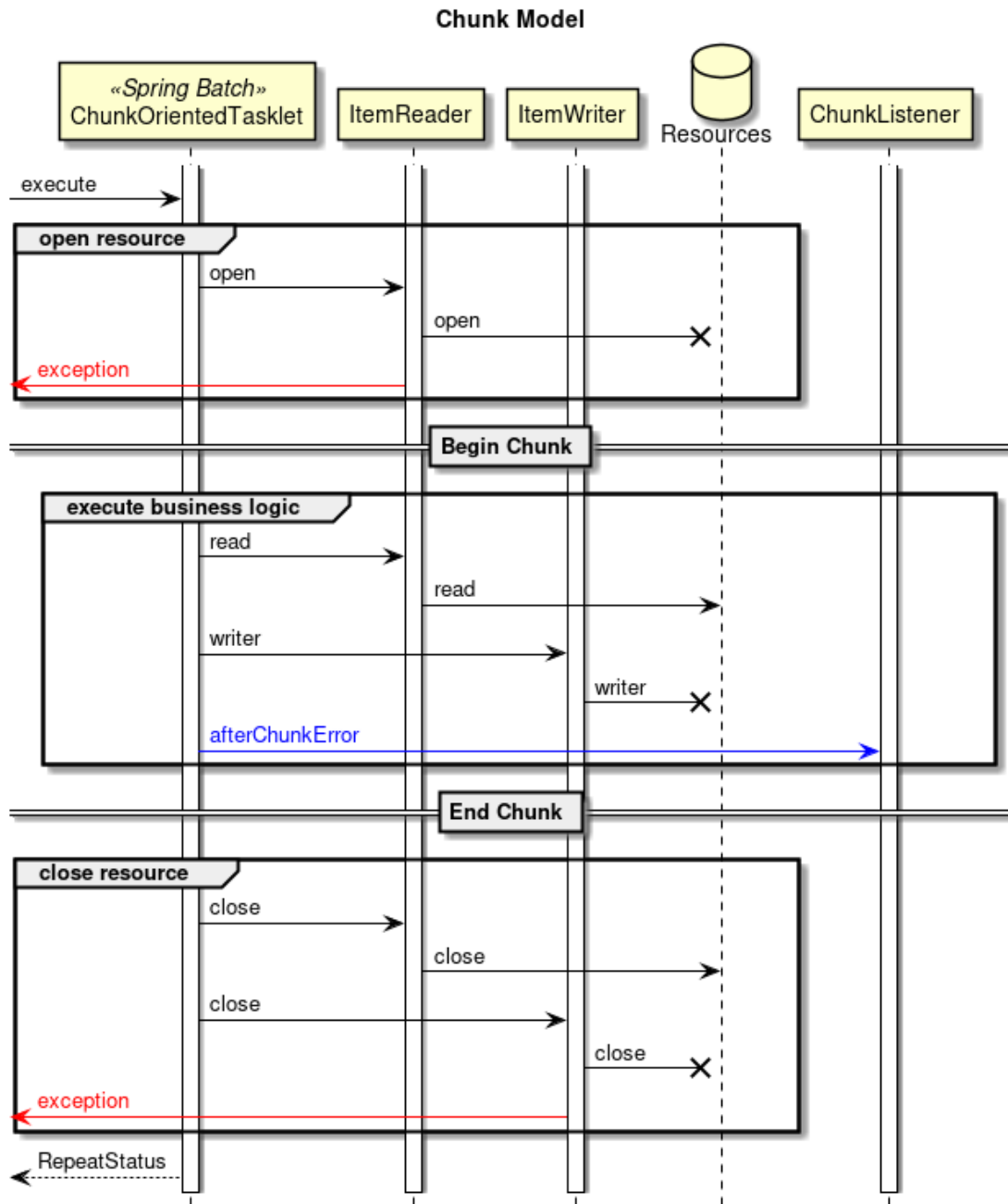
図 44. チャンクモデルでの例外ハンドリング概略図
