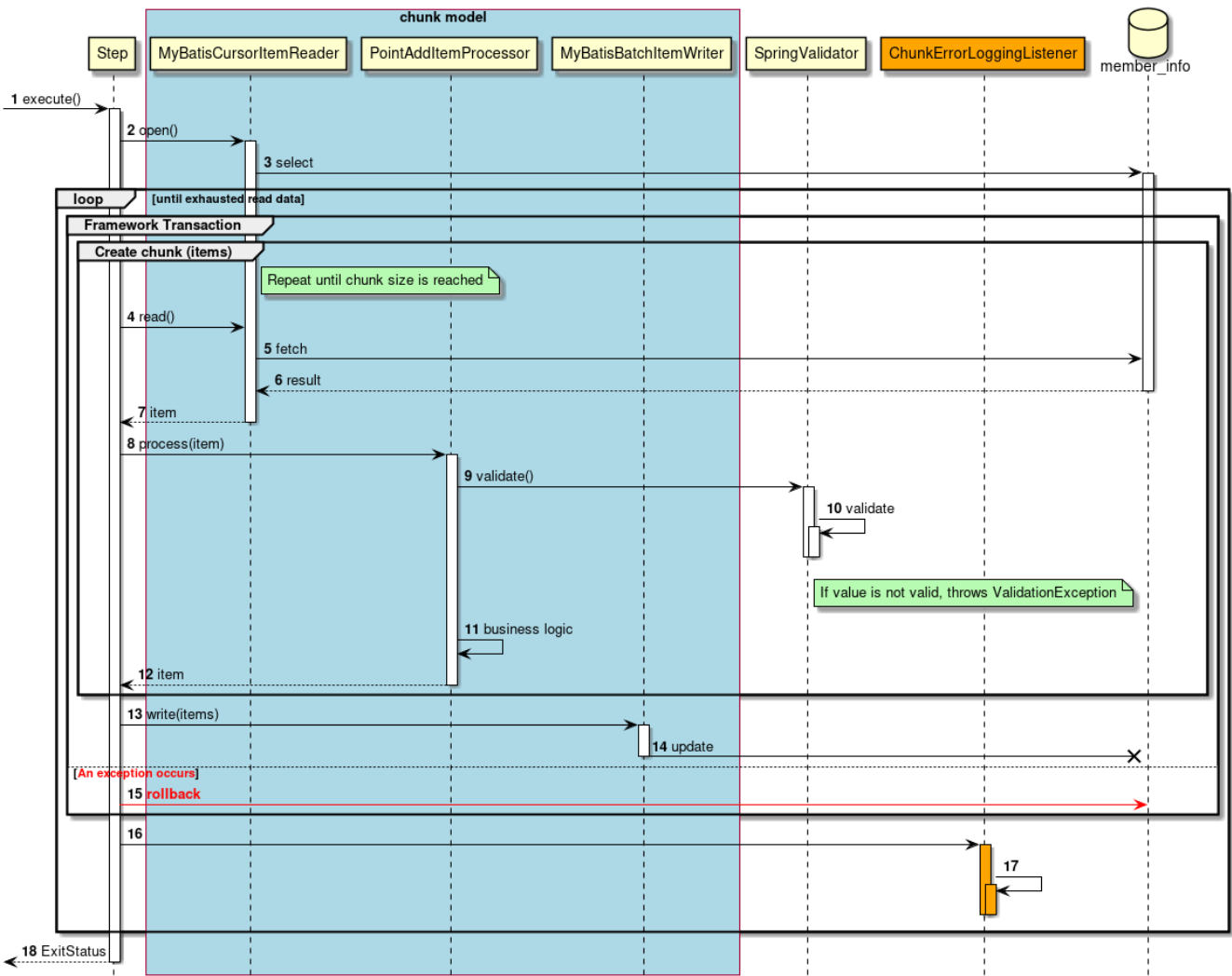
図 101. チャンクモデルのシーケンス図
