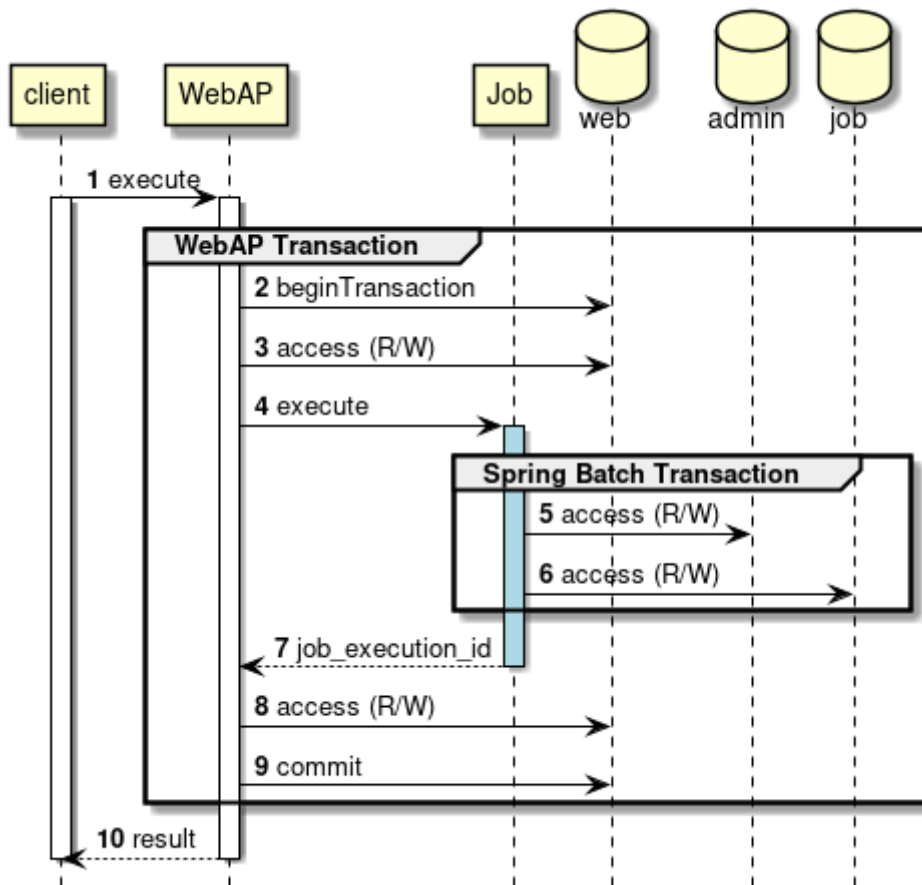
図 33. WebAPサーバ処理のトランザクション
