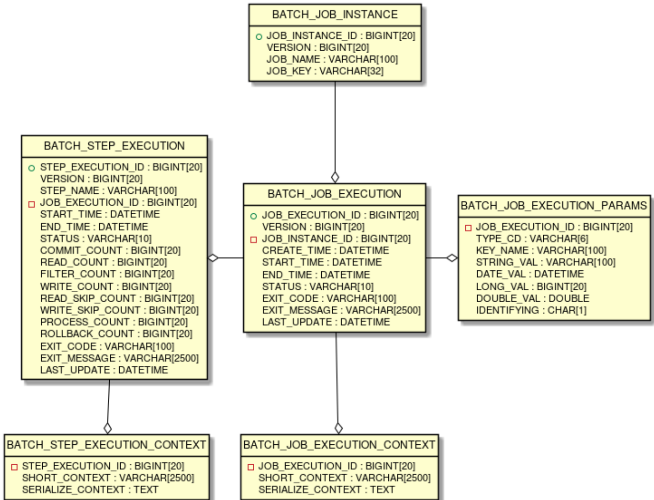
図 8. ER図
