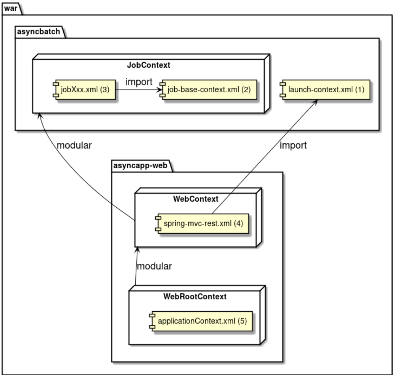
図 21. ApplicationContextの構成
