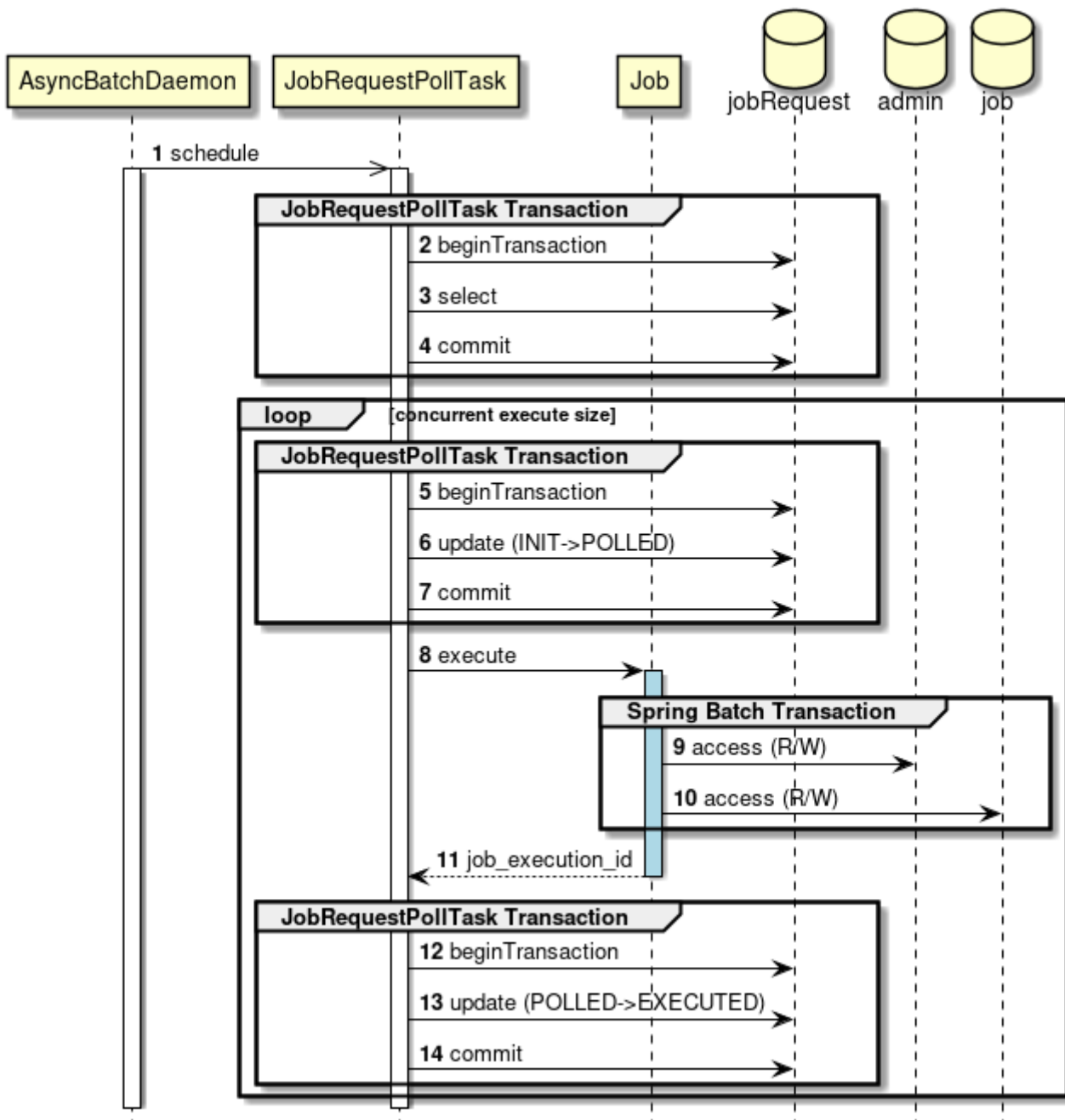
図 32. DBポーリング処理のトランザクション
