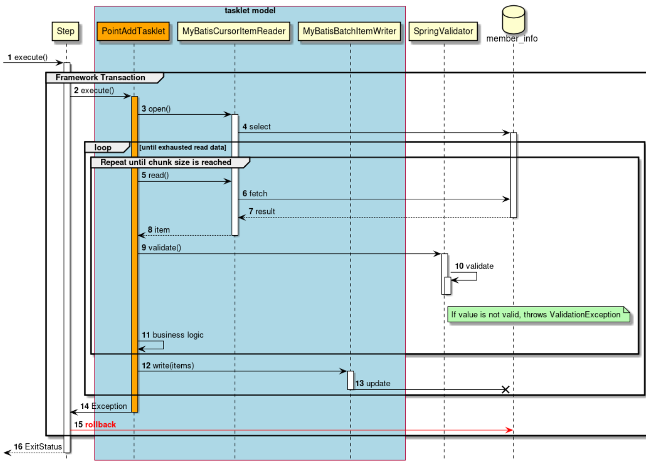
図 94. タスクレットモデルのシーケンス図
