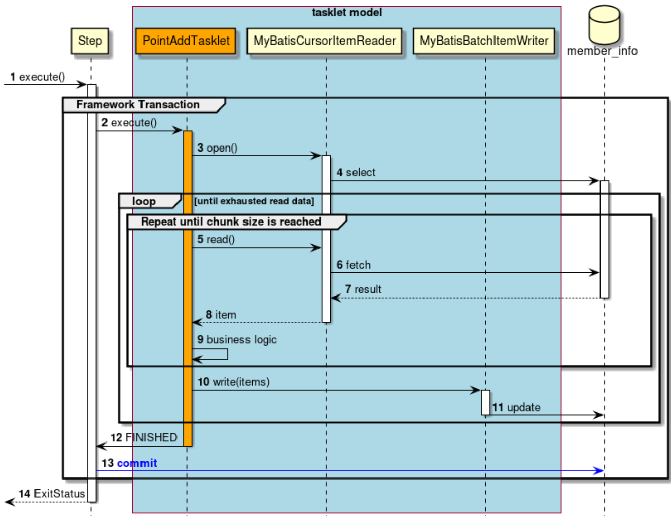
図 80. タスクレットモデルのシーケンス図
