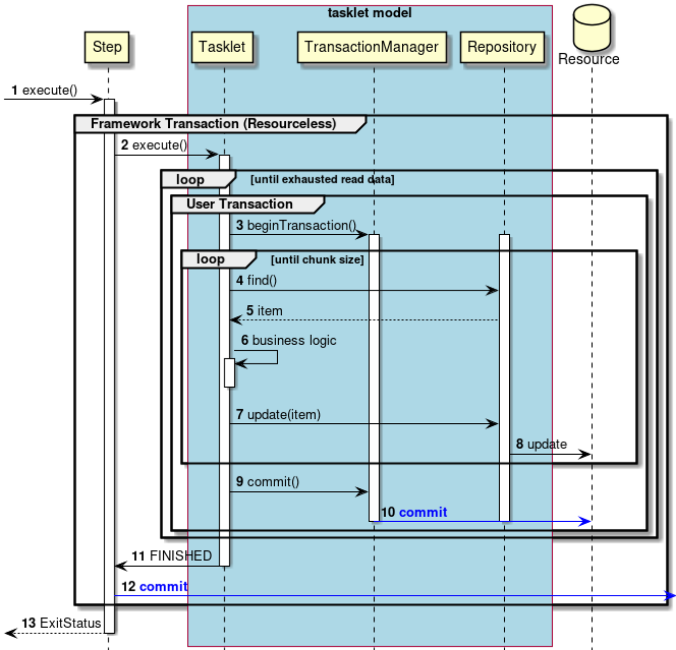
図 30. 正常系のシーケンス図
