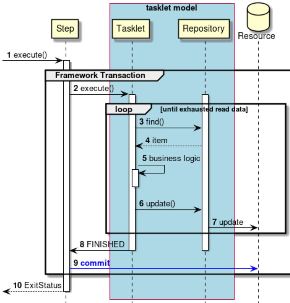
図 28. 正常系のシーケンス図
