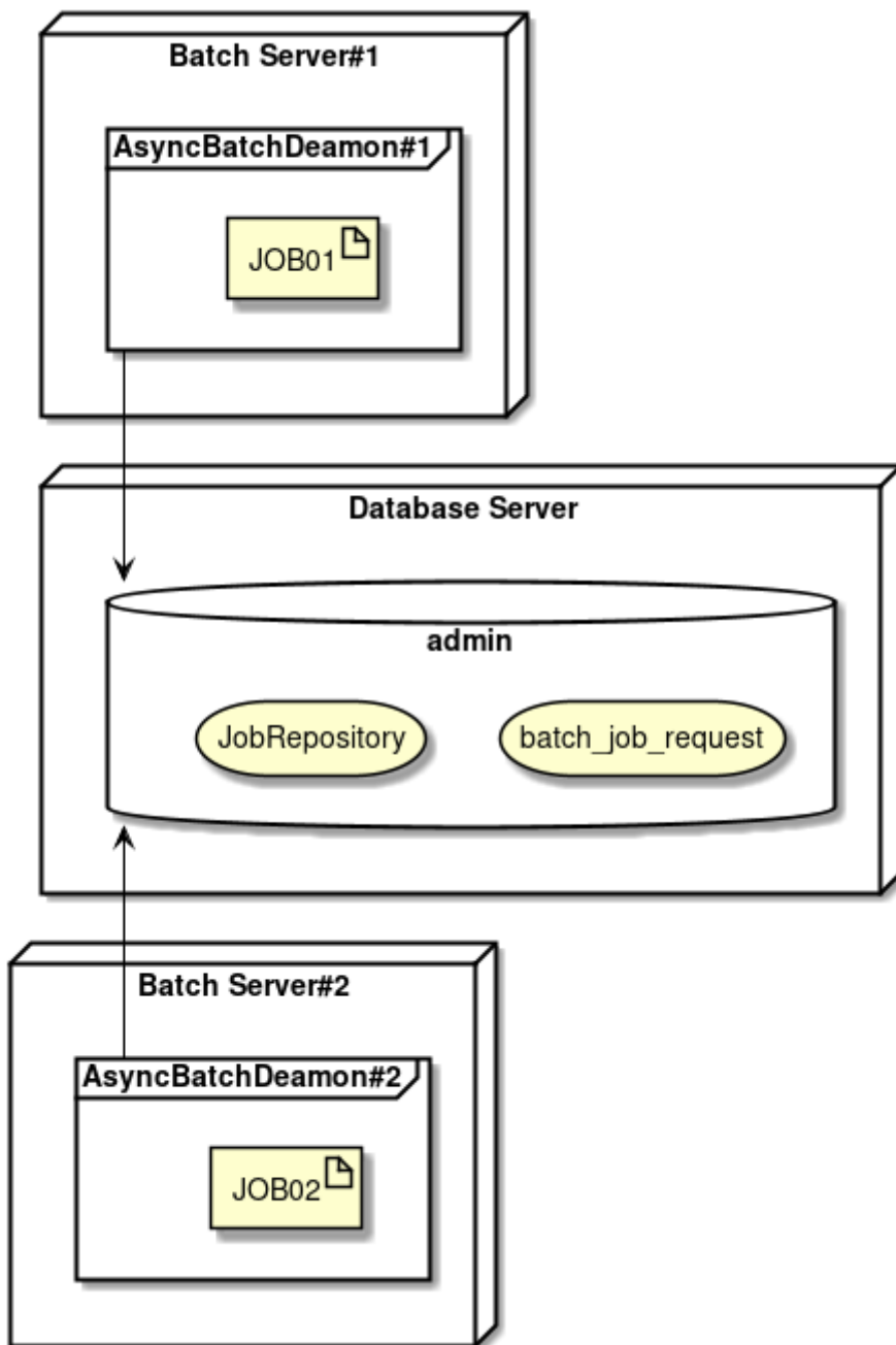
図 19. 複数起動の概略図
