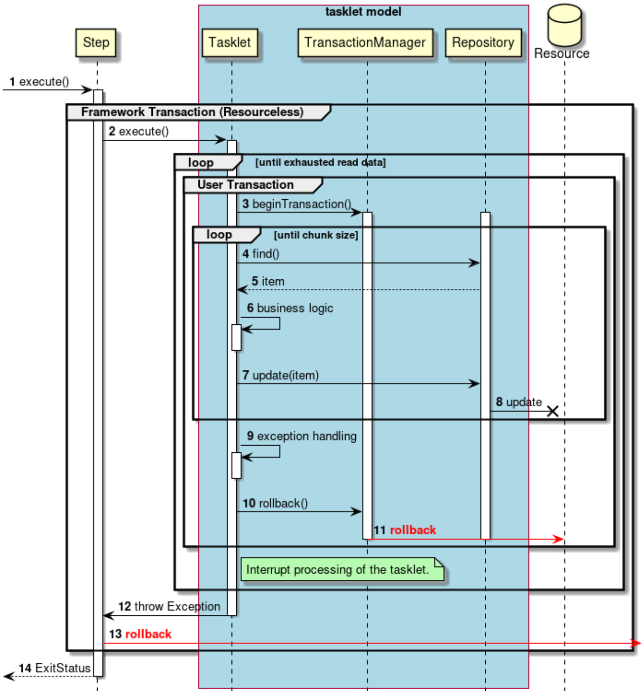
図 31. 異常系のシーケンス図
