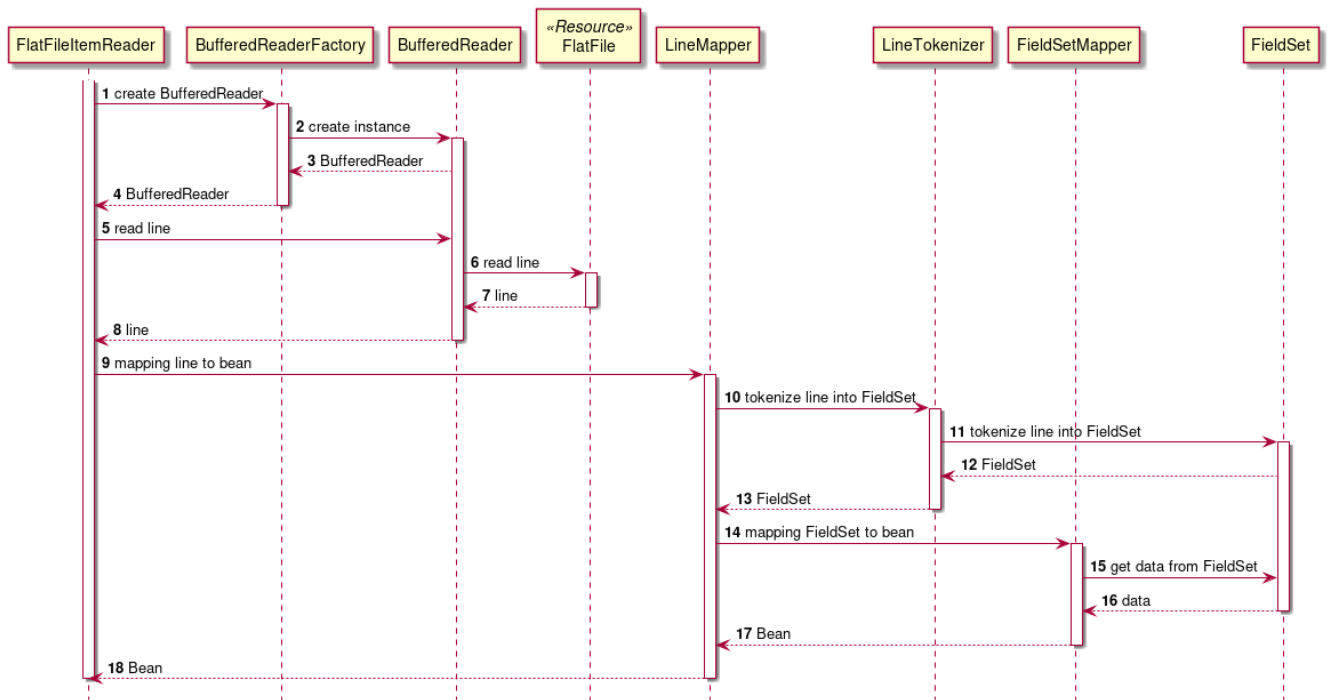
図 37. 各コンポーネントの呼び出し関係
