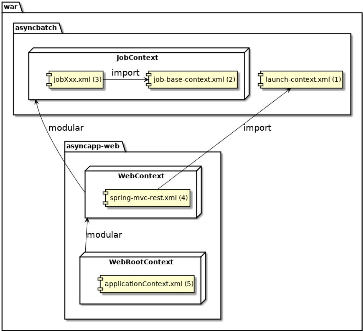
図 21. ApplicationContextの構成
