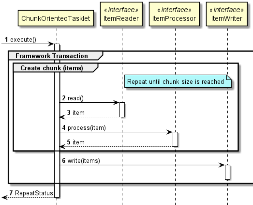
図 7. ChunkOrientedTasklet によるチャンク処理
