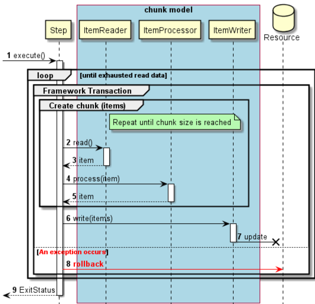
図 27. 異常系のシーケンス図
