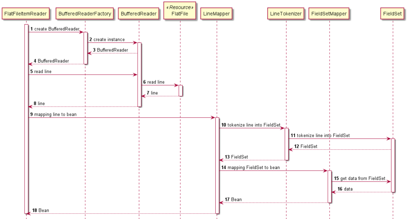
図 37. 各コンポーネントの呼び出し関係
