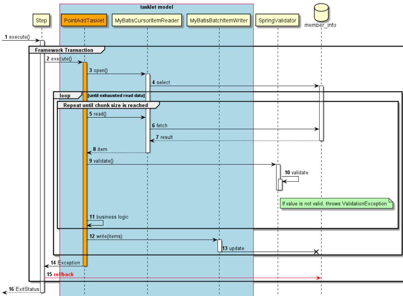
図 93. タスクレットモデルのシーケンス図
