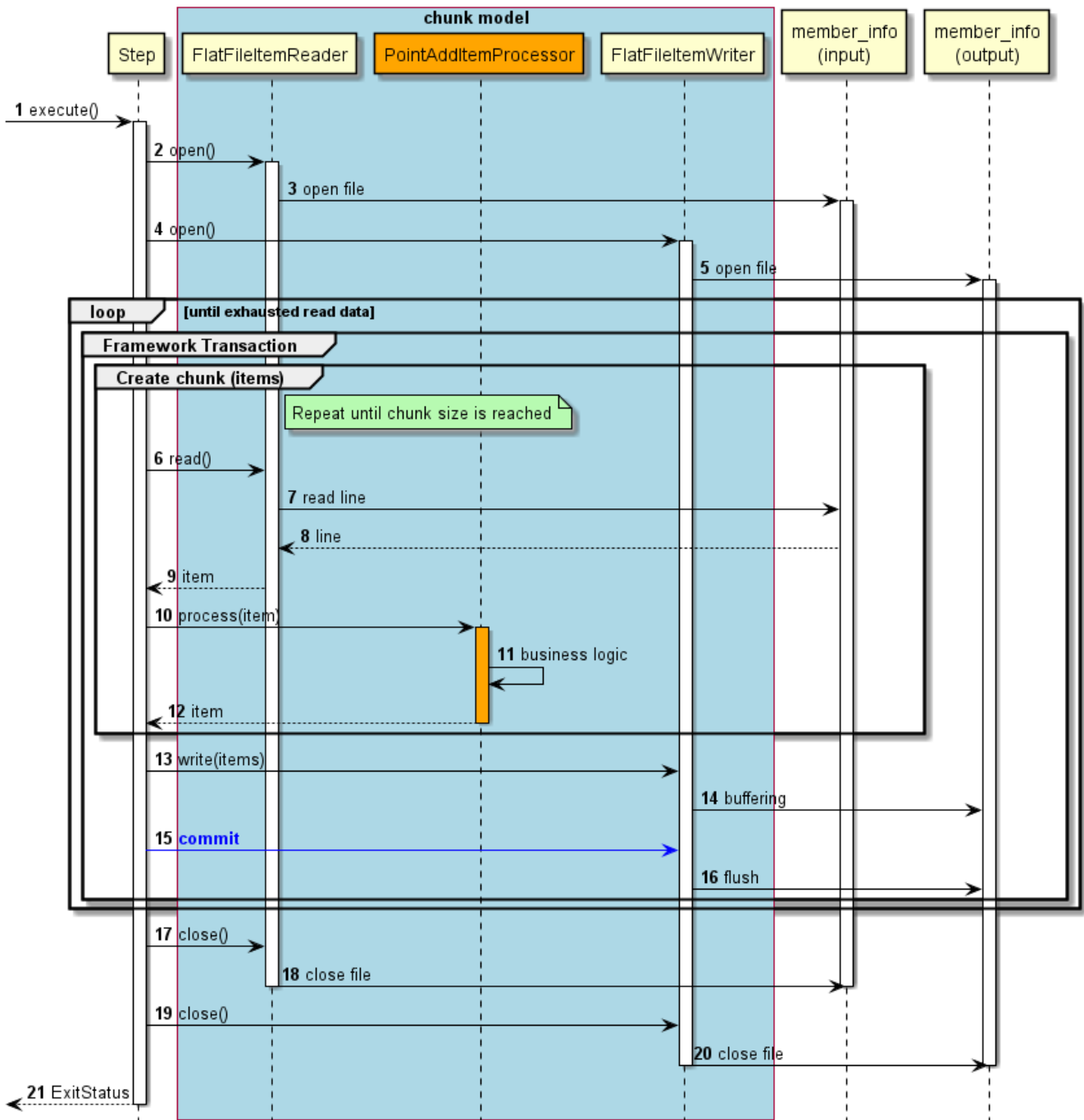
図 85. チャンクモデルのシーケンス図
