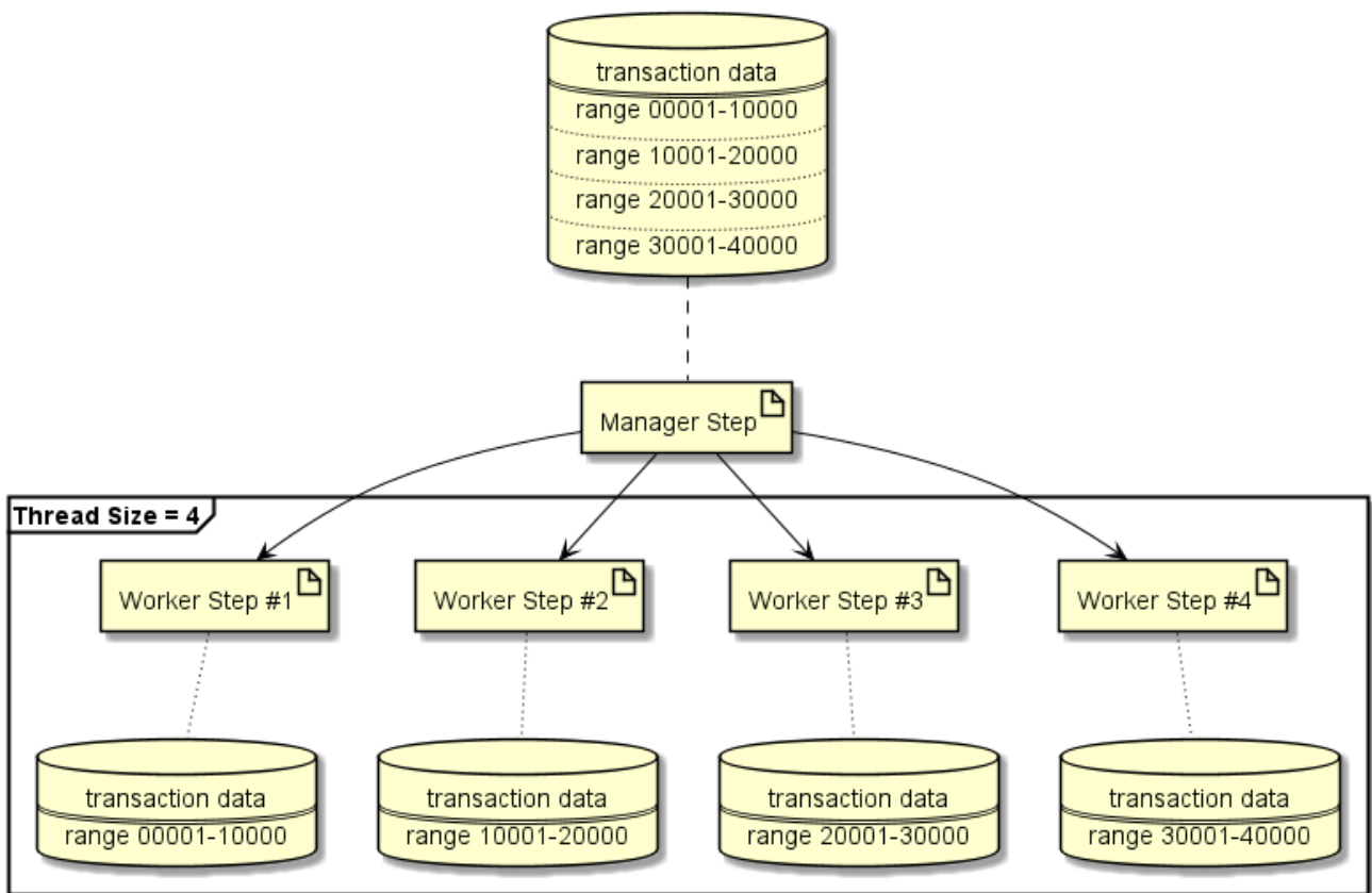
図 54. 処理イメージ図
