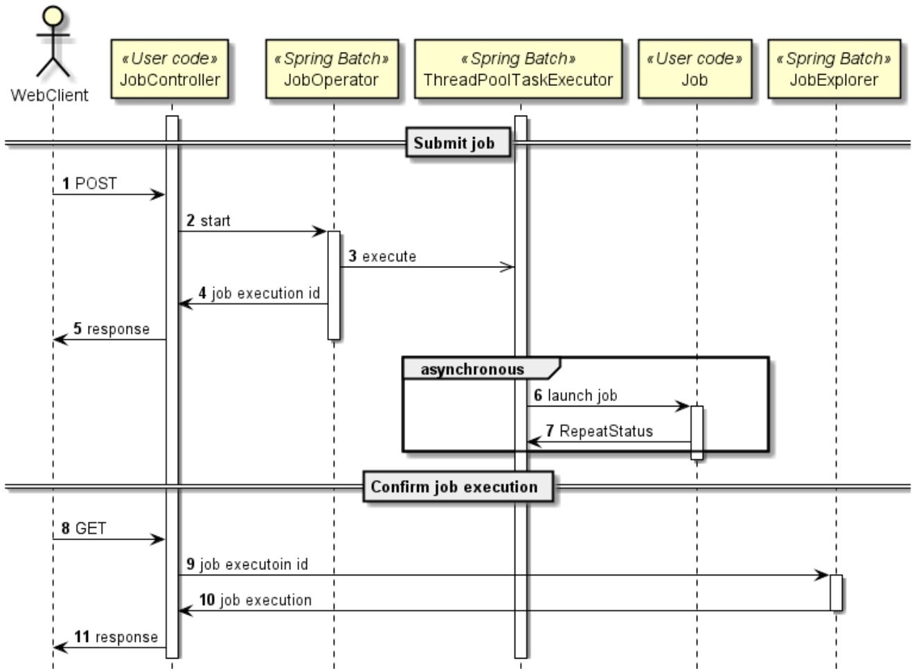
図 20. 非同期実行(Webコンテナ)のシーケンス図
