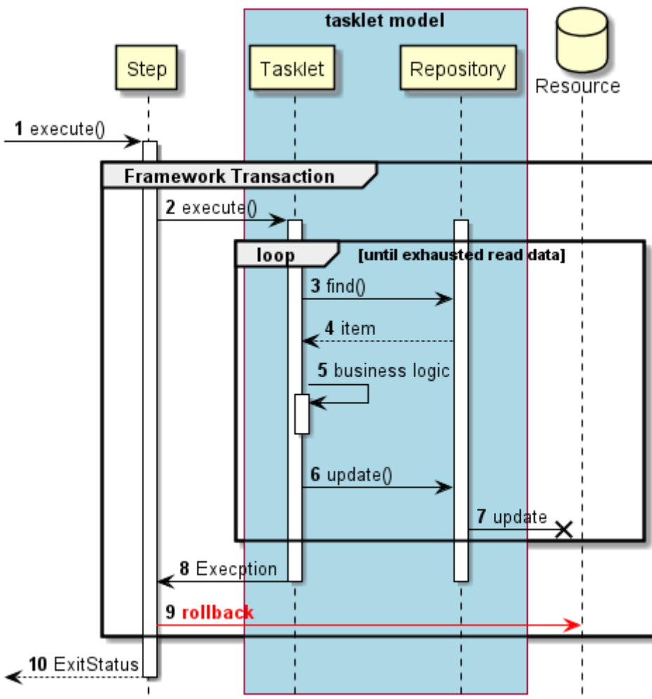
図 29. 異常系のシーケンス図
