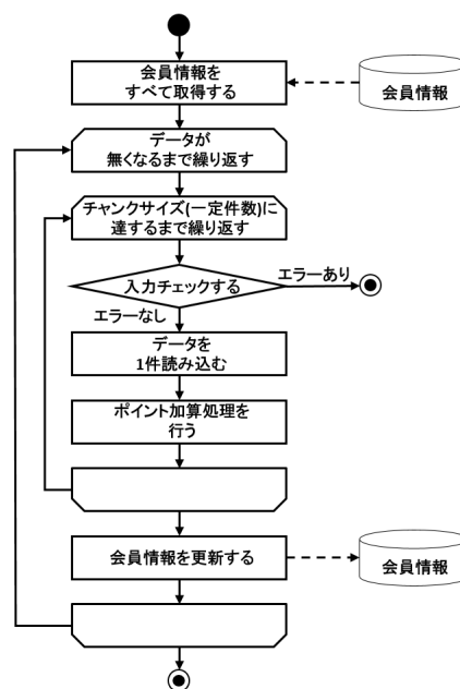
図 91. 入力データの妥当性検証を行うジョブの処理フロー
