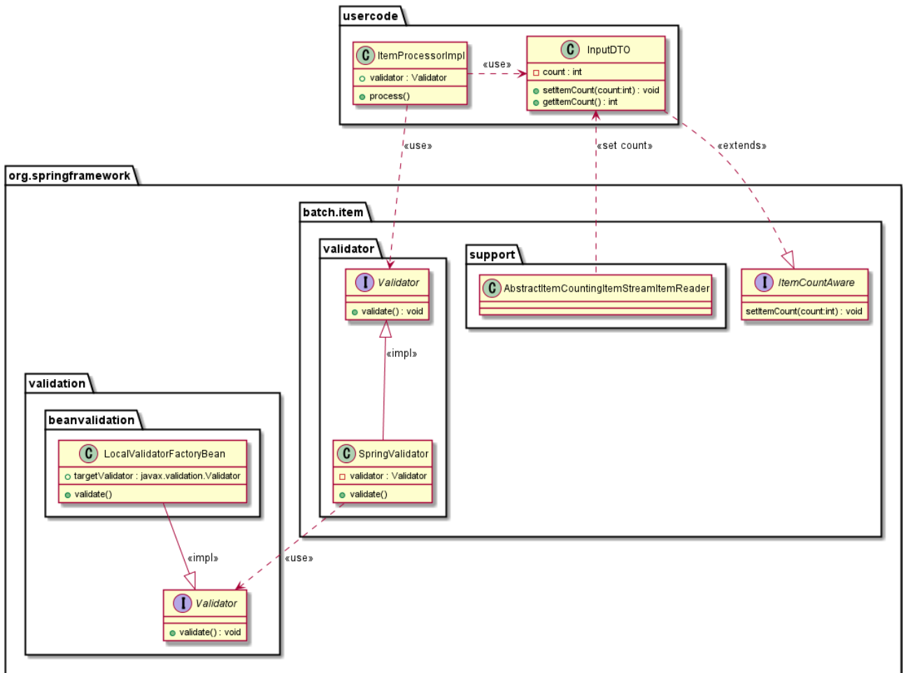
図 43. 入力チェックの関連クラス
