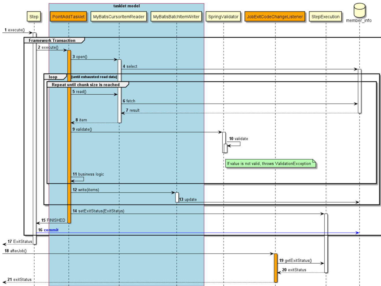
図 109. タスクレットモデルの処理シーケンス図
