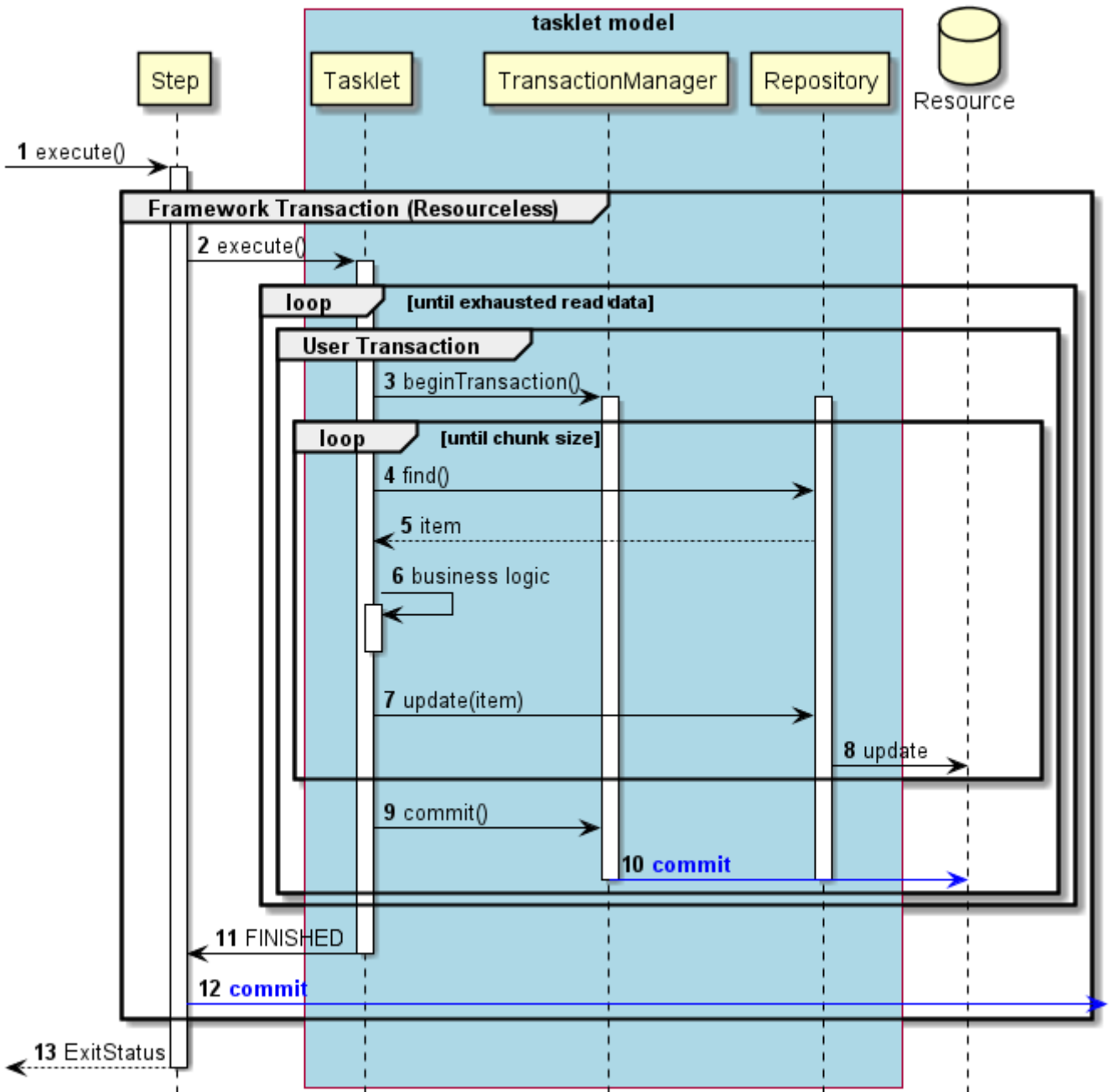
図 30. 正常系のシーケンス図
