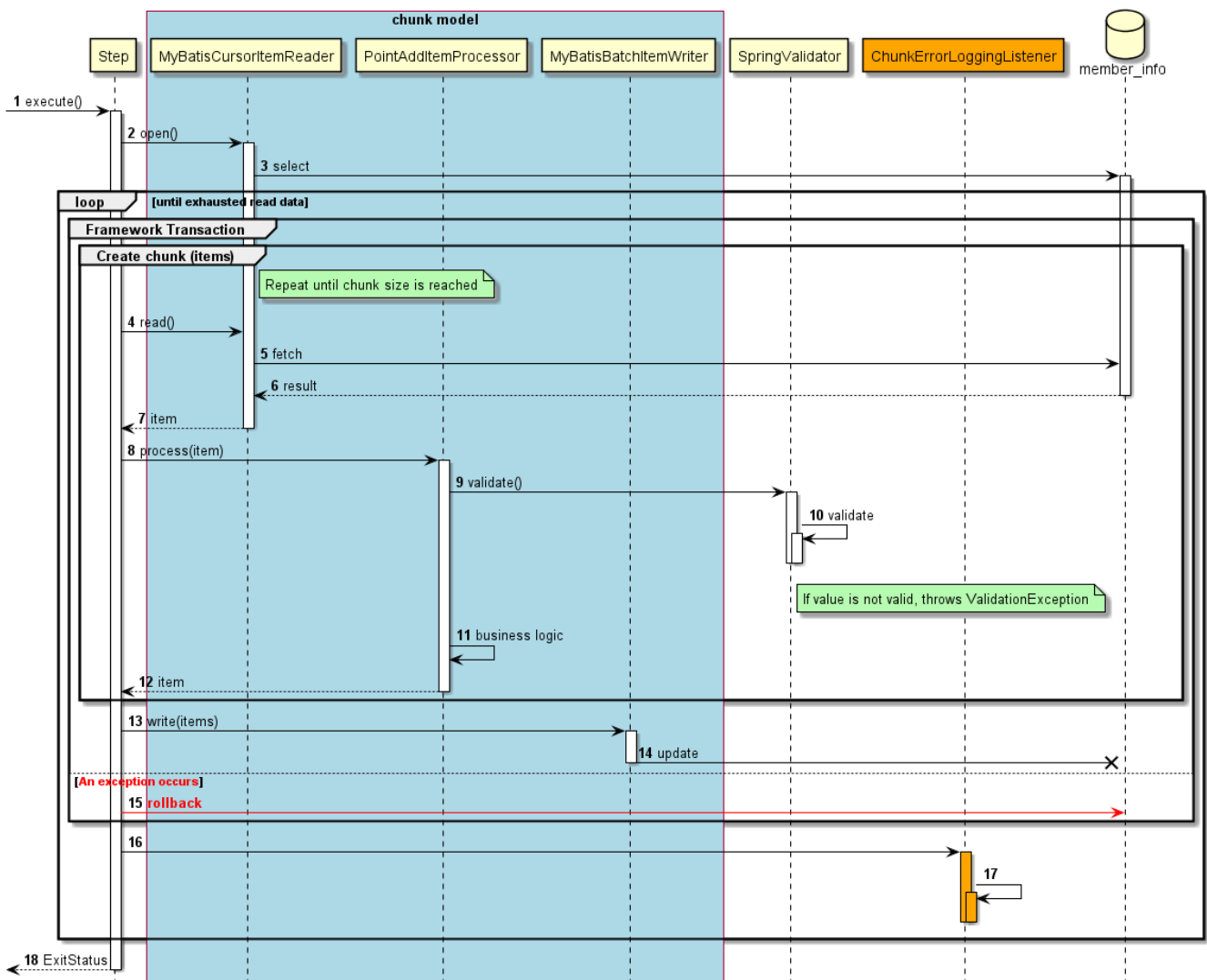
図 100. チャンクモデルのシーケンス図
