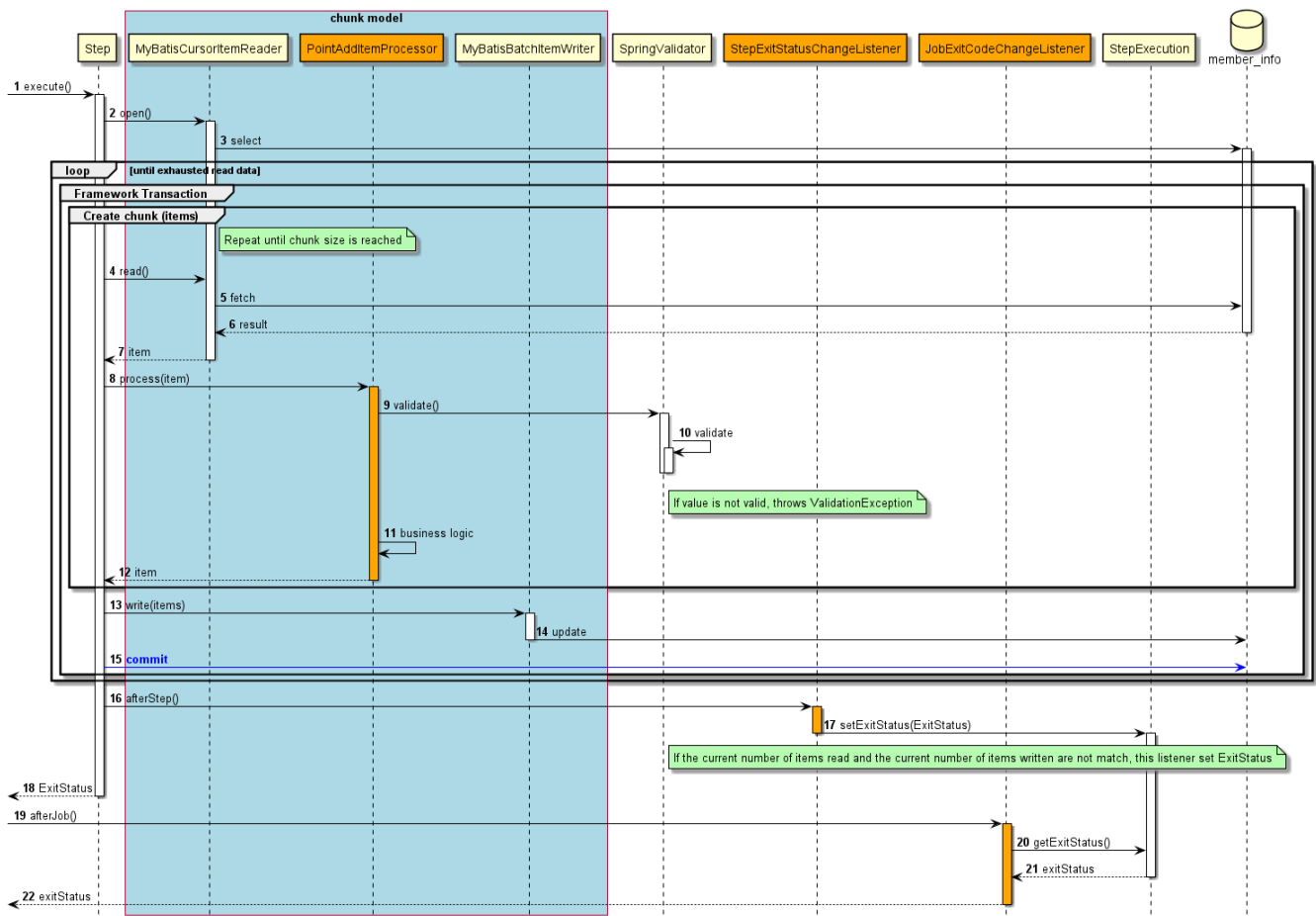
図 108. チャンクモデルのシーケンス図
