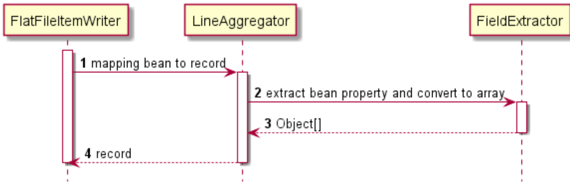
図 39. 各コンポーネントの呼び出し関係
