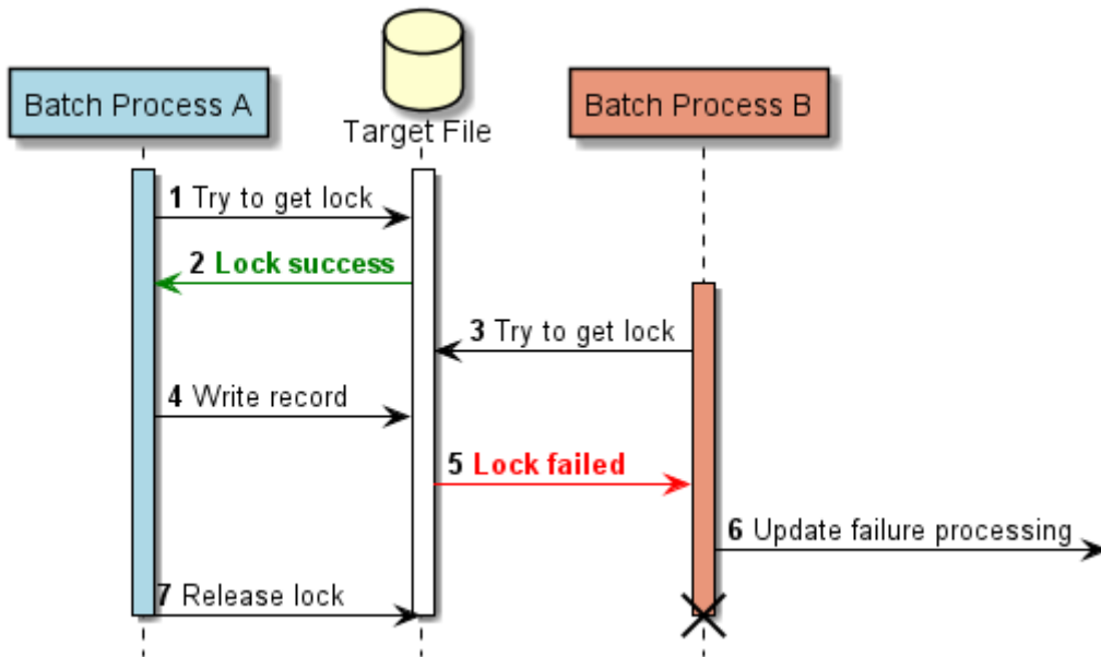
図 41. ファイルロックの実施イメージ
