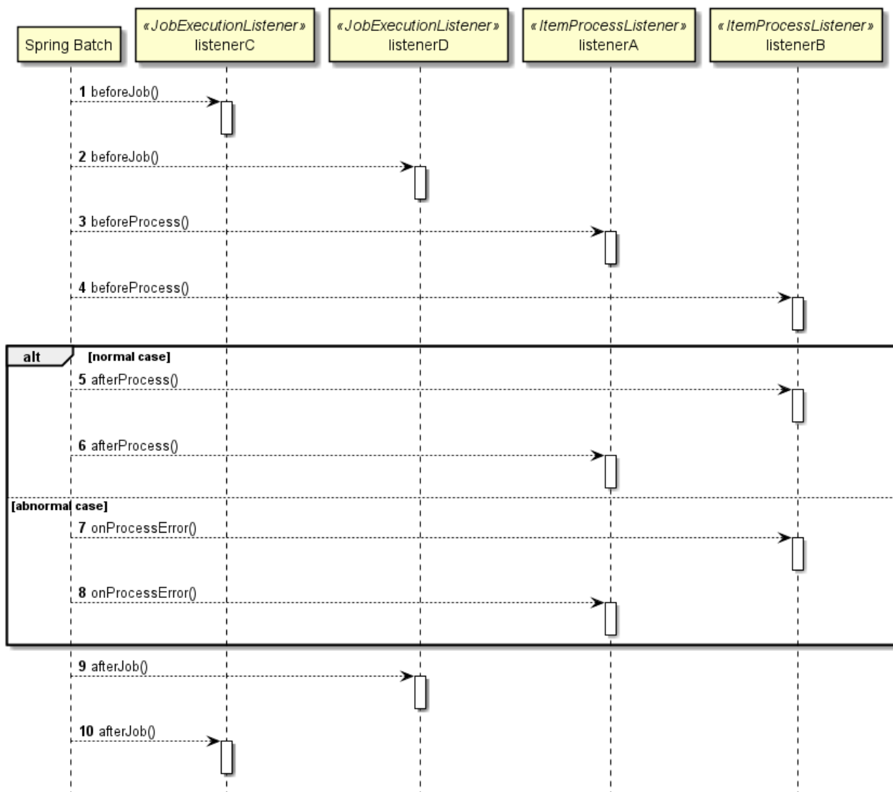
図 25. リスナーの起動順序
