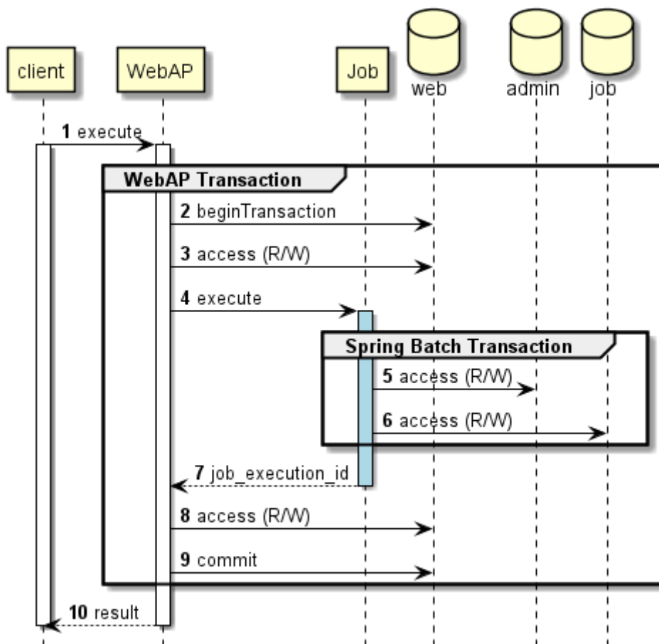
図 33. WebAPサーバ処理のトランザクション
