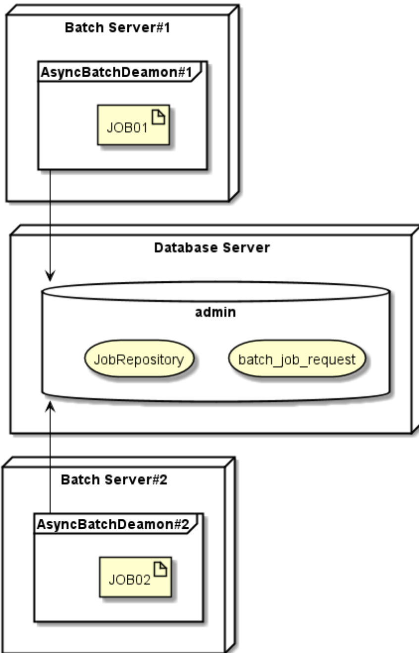
図 19. 複数起動の概略図
