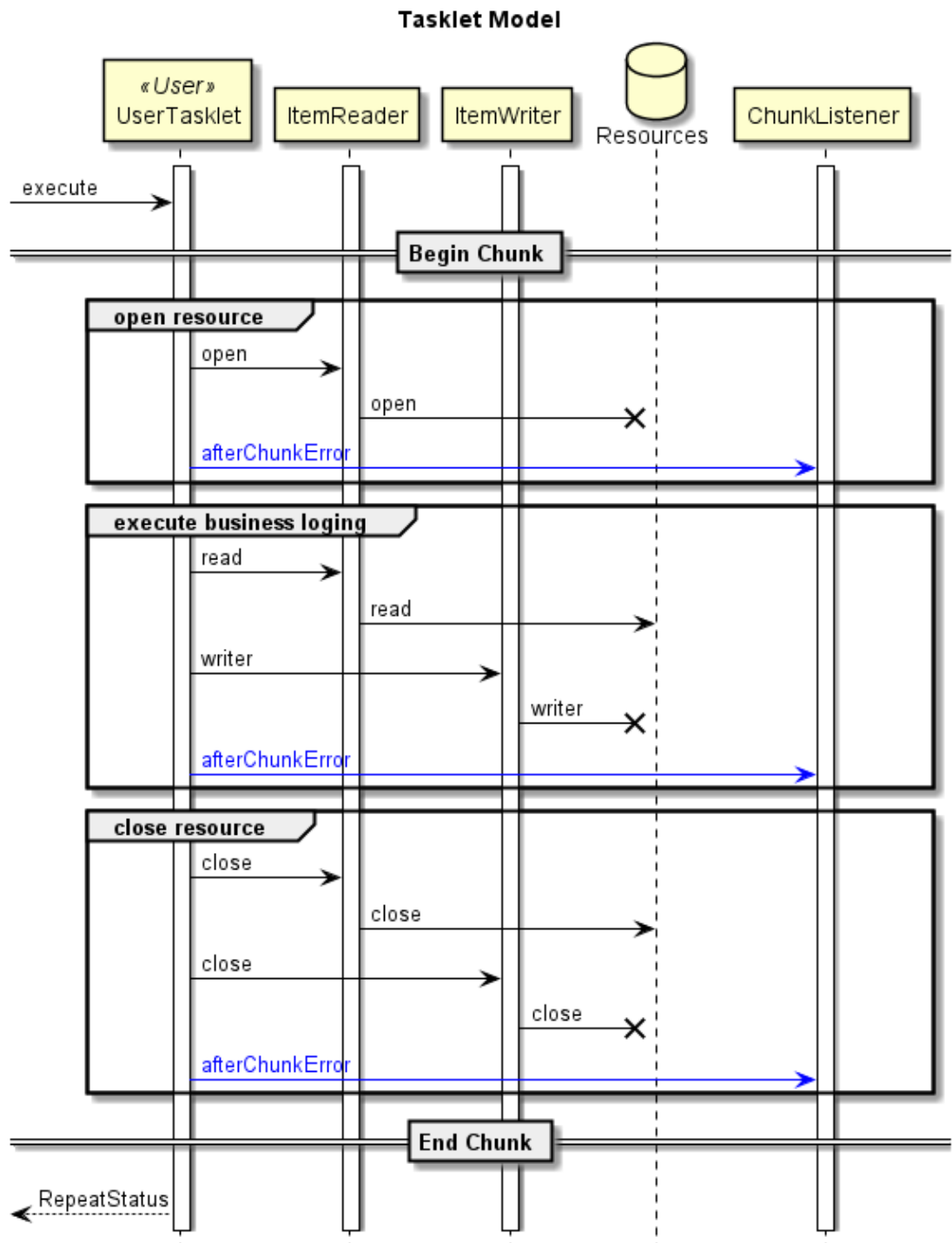
図 45. タスクレットモデルでの例外ハンドリング概略図
