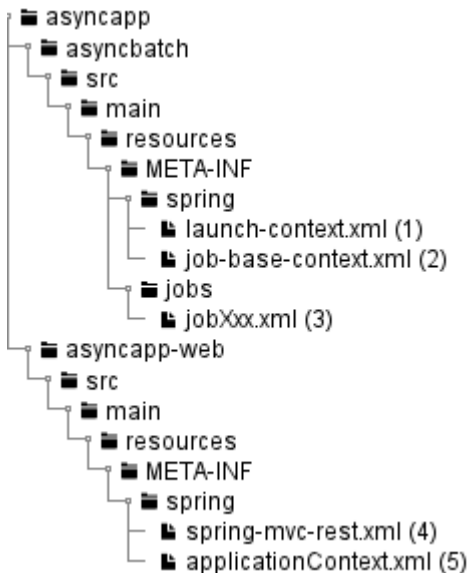
図 22. Bean定義ファイルの構成
