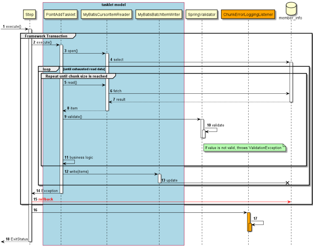
図 101. タスクレットモデルのシーケンス図
