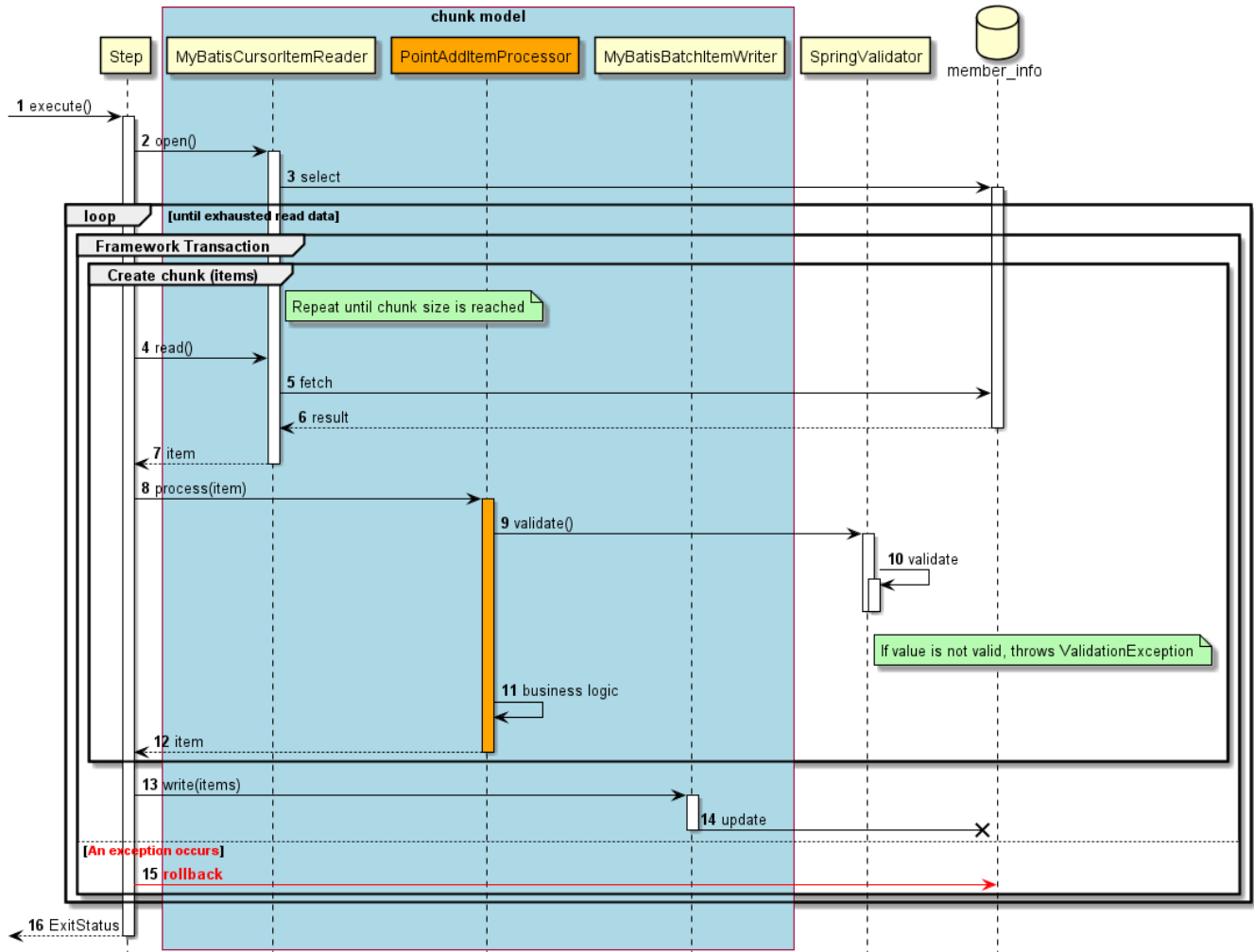
図 92. チャンクモデルのシーケンス図
