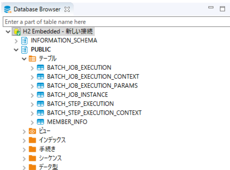
図 75. Show Tables
