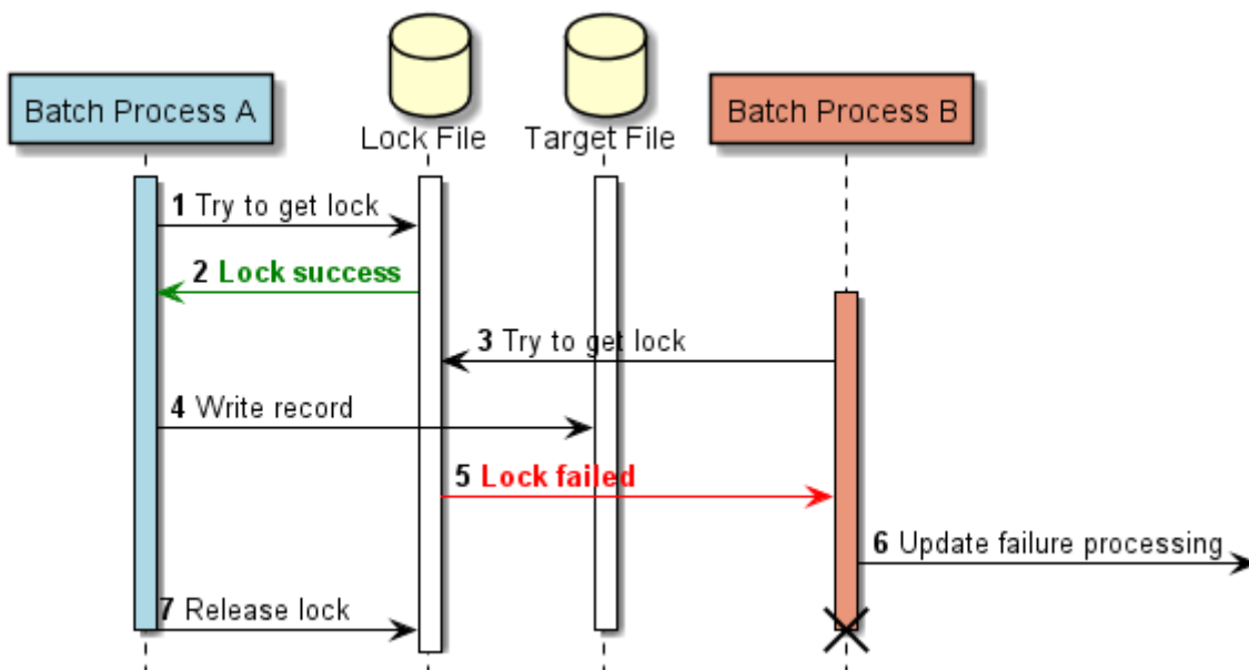
図 42. ロック用ファイルを用いたファイルロックの実施イメージ
