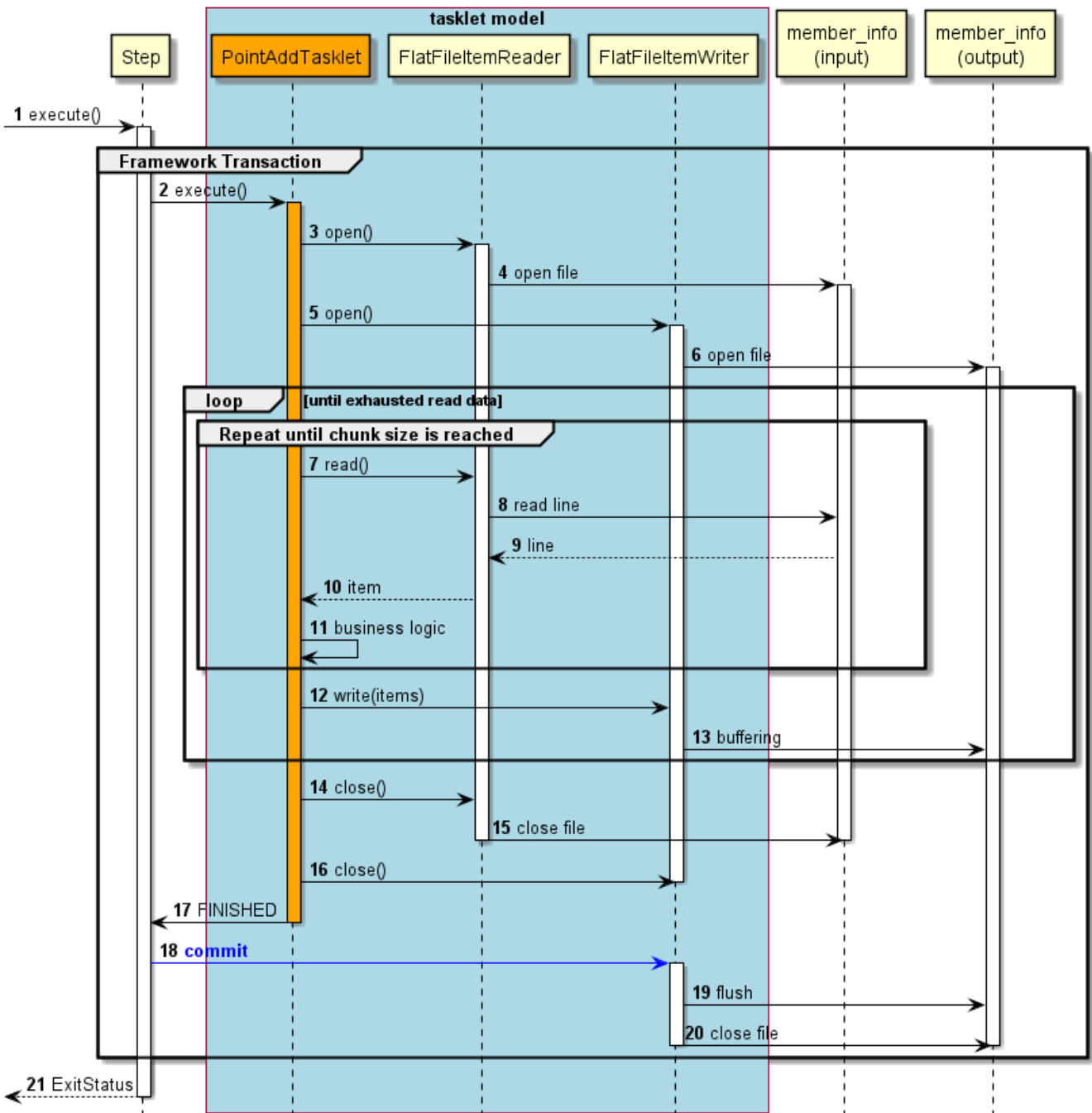
図 86. タスクレットモデルのシーケンス図
