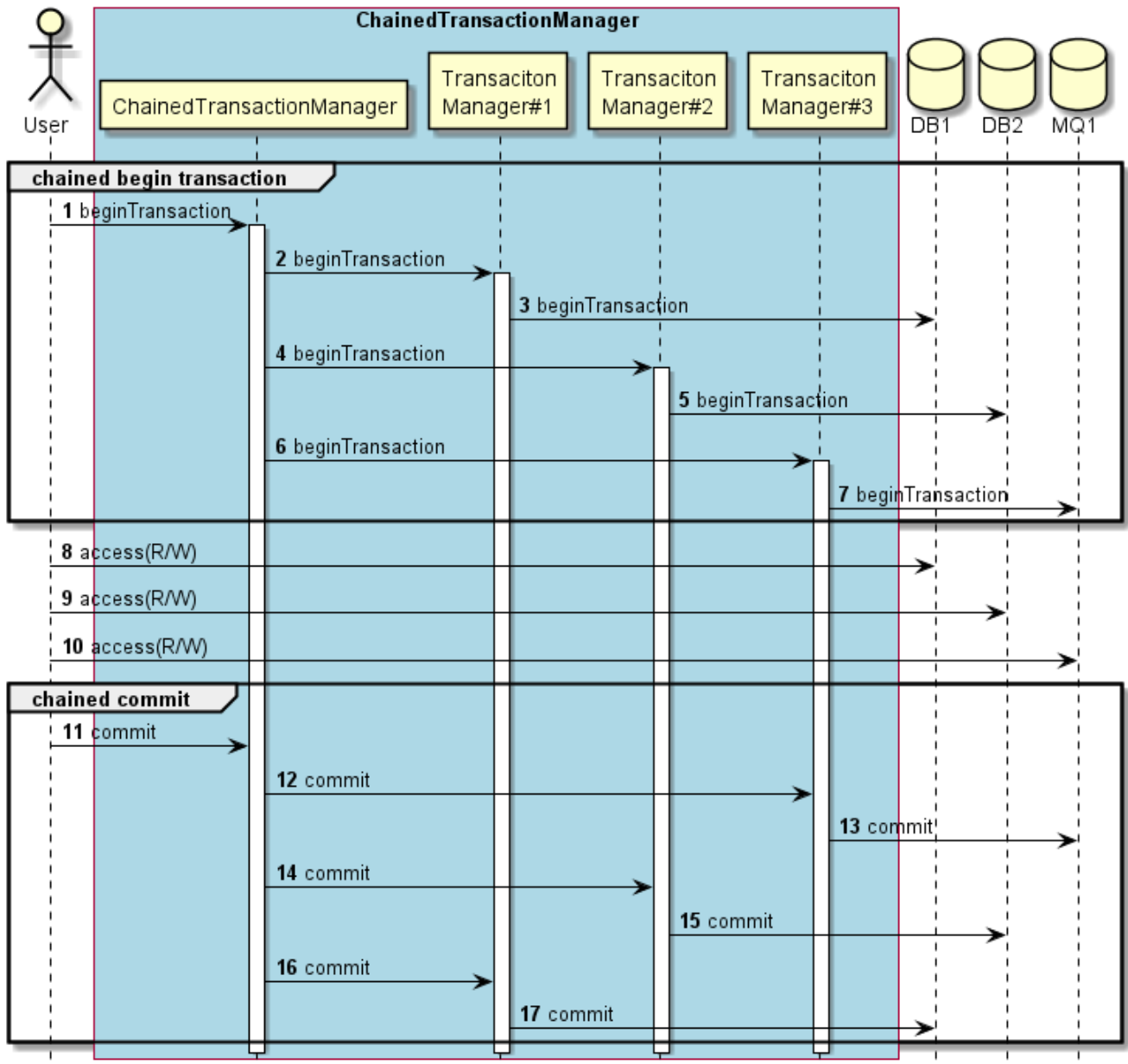
図 34. Best Efforts 1PC パターンの概念図
