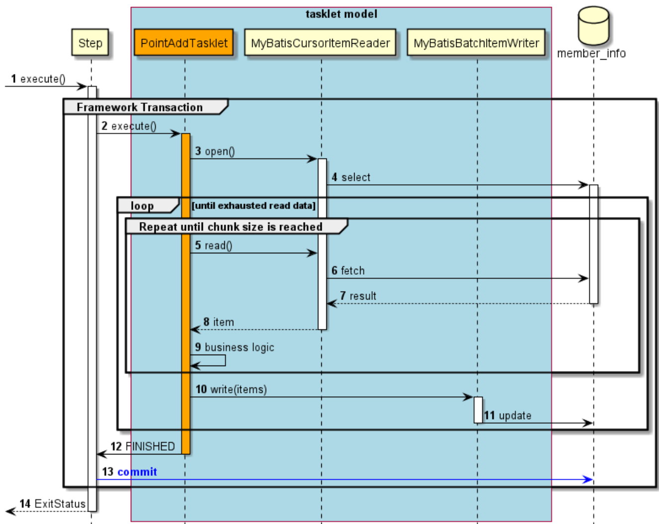
図 79. タスクレットモデルのシーケンス図
