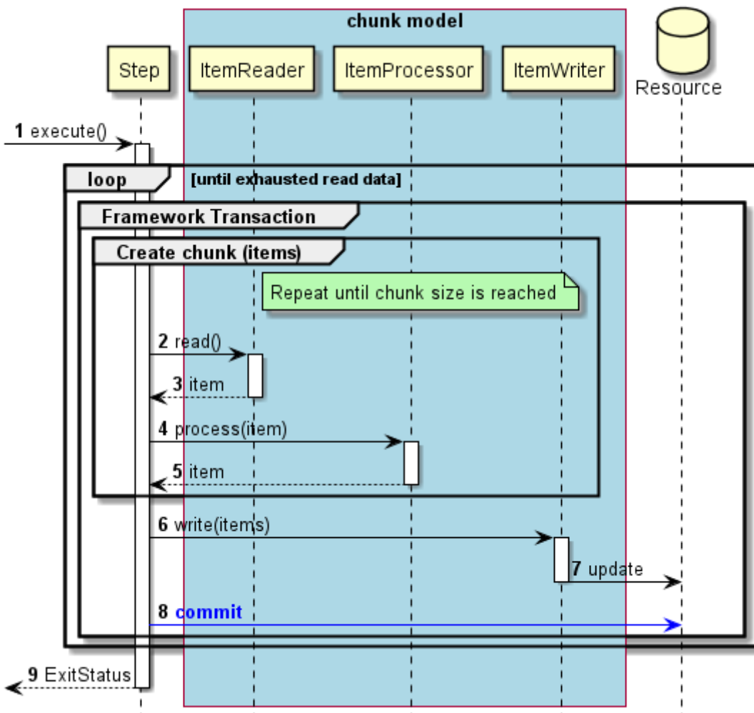
図 26. 正常系のシーケンス図
