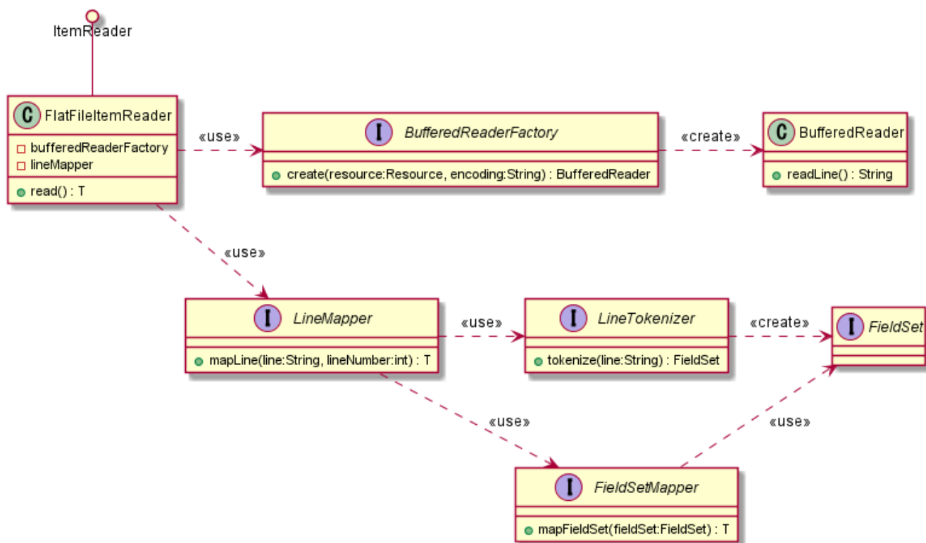
図 36. フラットファイルの入力を行うために使用するクラスの関連
