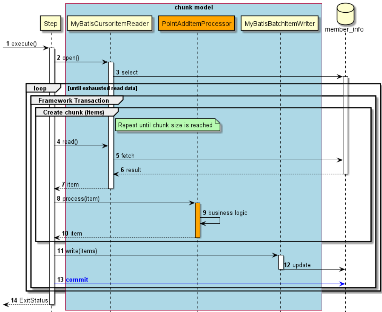
図 78. チャンクモデルのシーケンス図
