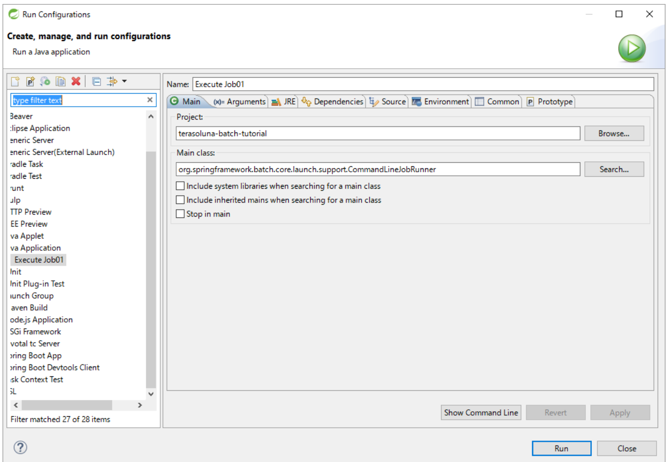
図 70. Run Job01
