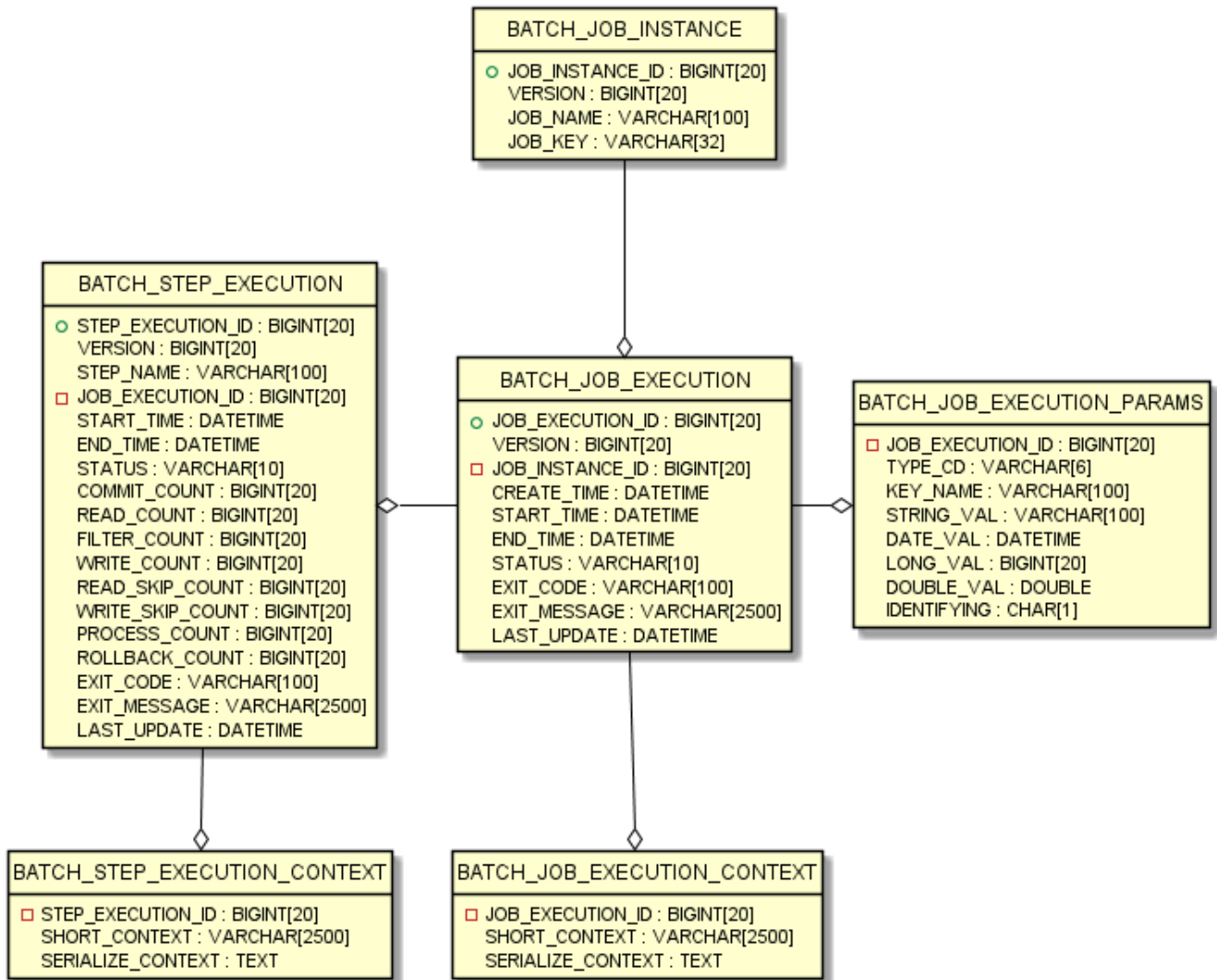
図 8. ER図
