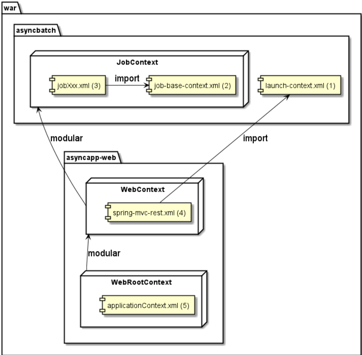
図 21. ApplicationContextの構成
