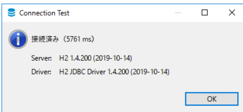
図 67. Connection Test
