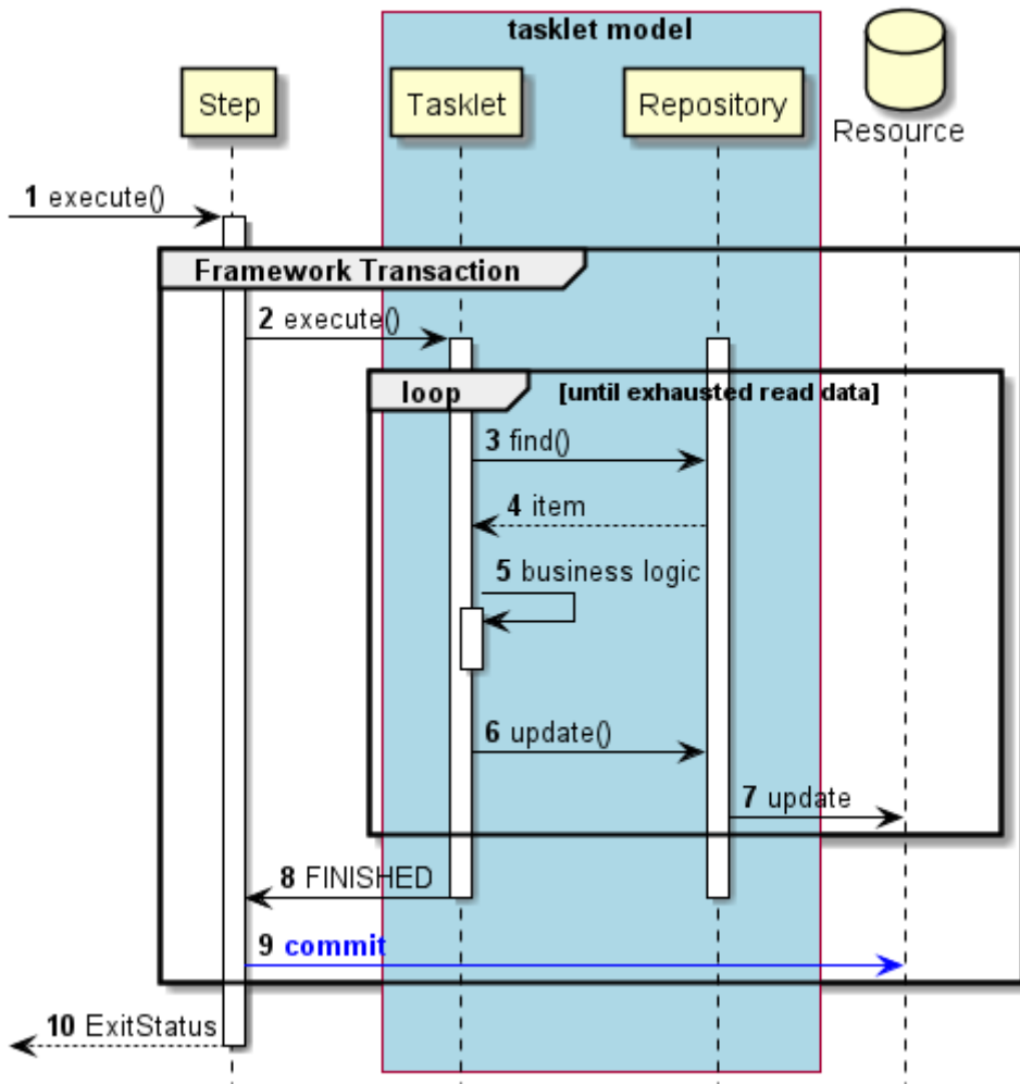
図 28. 正常系のシーケンス図
